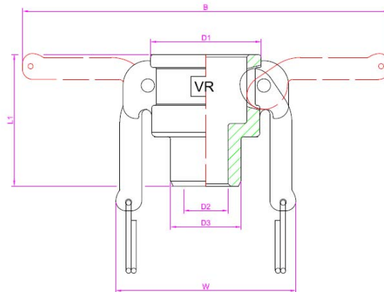
Raccordo Rapido FEMMINA filettato Maschio Coupling female threaded Male
